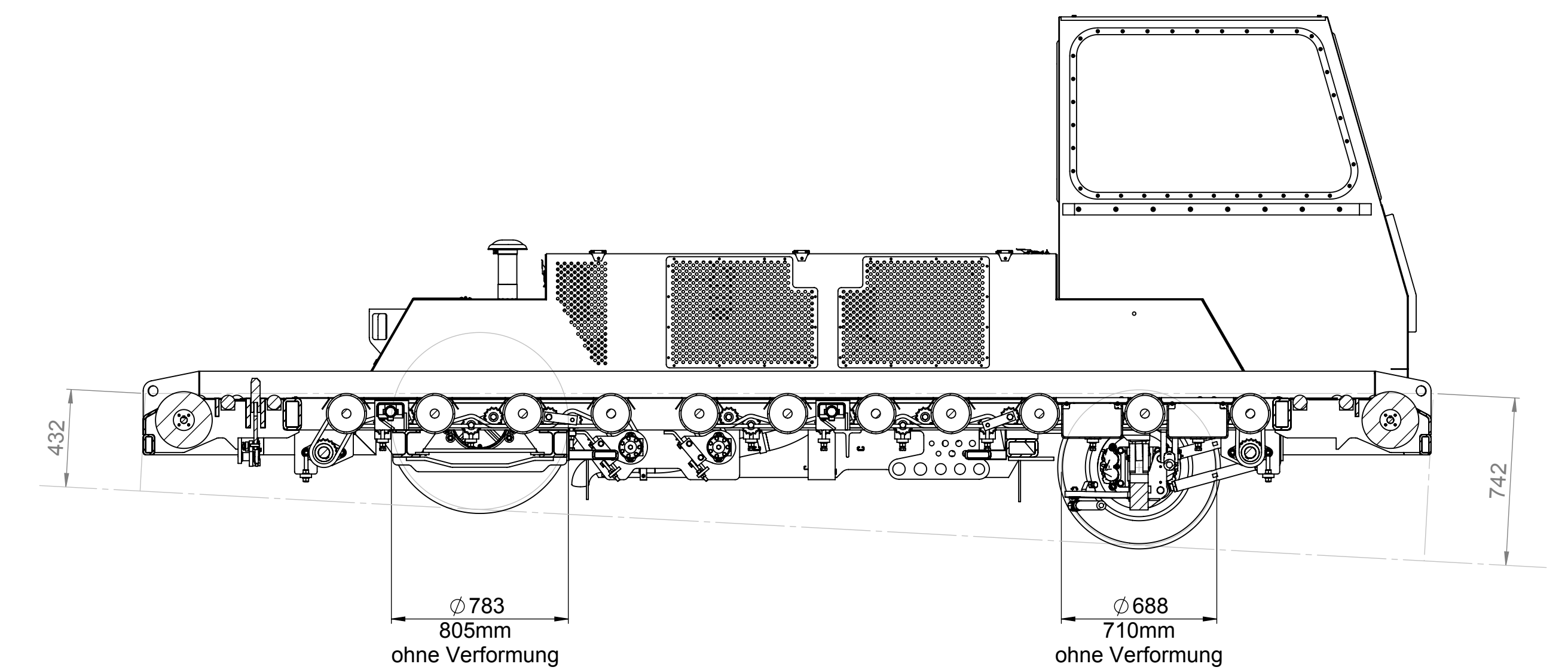
SCHNITT C-C Messung erfolgt über OK-Stahlrollen
