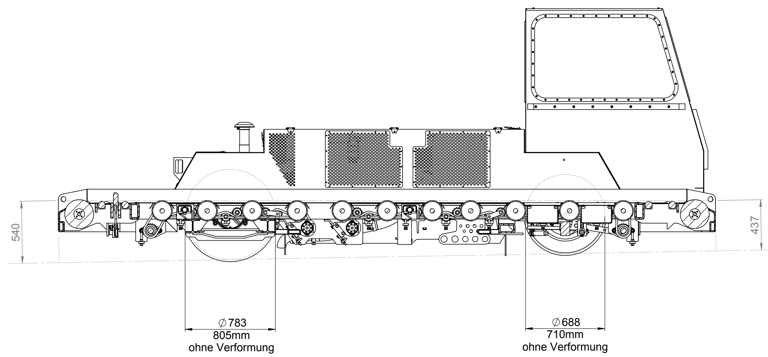
SCHNITT B-B Messung erfolgt über OK-Stahlrollen
