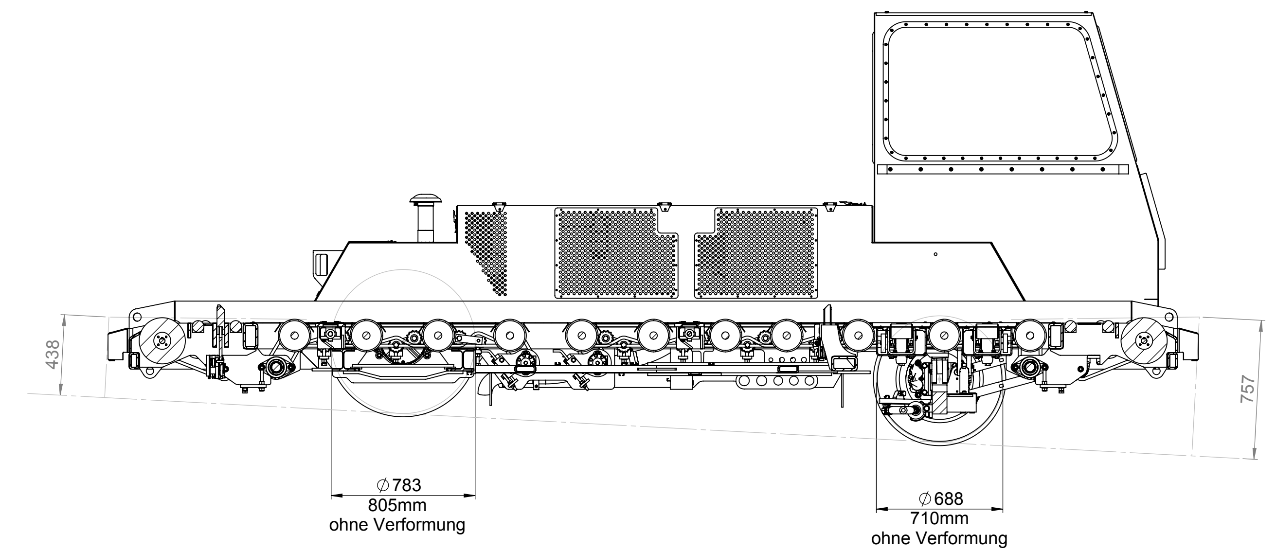
SCHNITT E-E Messung erfolgt über OK-Gummirolle
